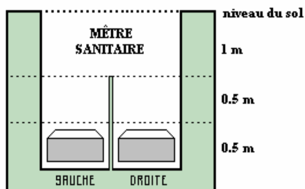
CAVEAU A CASES DOUBLES SEPARÉES PAR UN MUR DE REFEND
